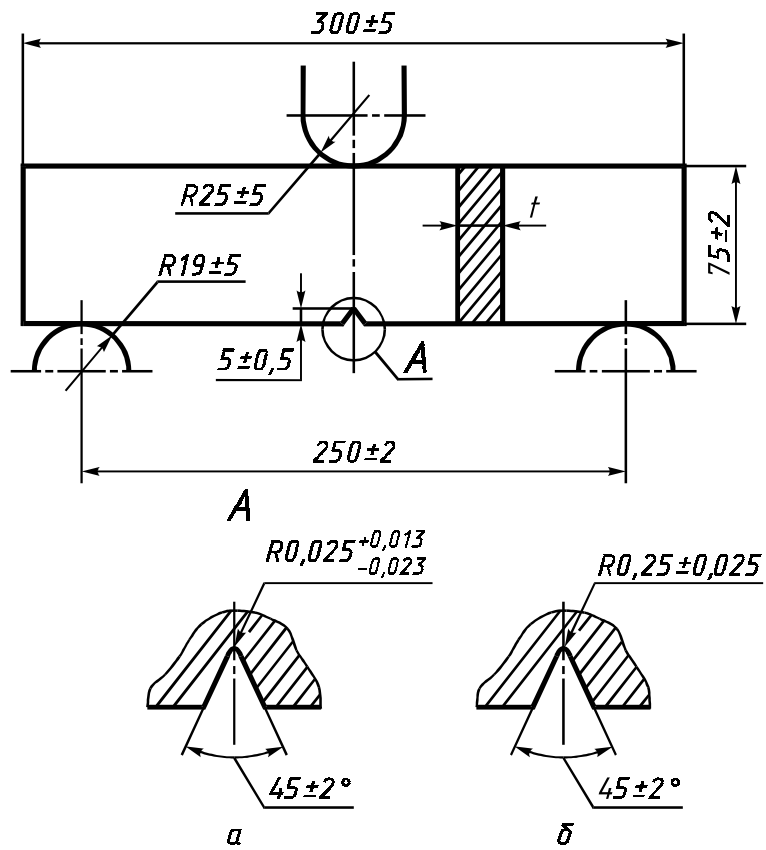
Рисунок 2 — Форма и размеры образца для ИПГ
