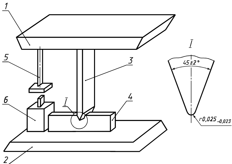
Рисунок 3 — Принципиальная схема приспособления для нанесения концентратора на образец
